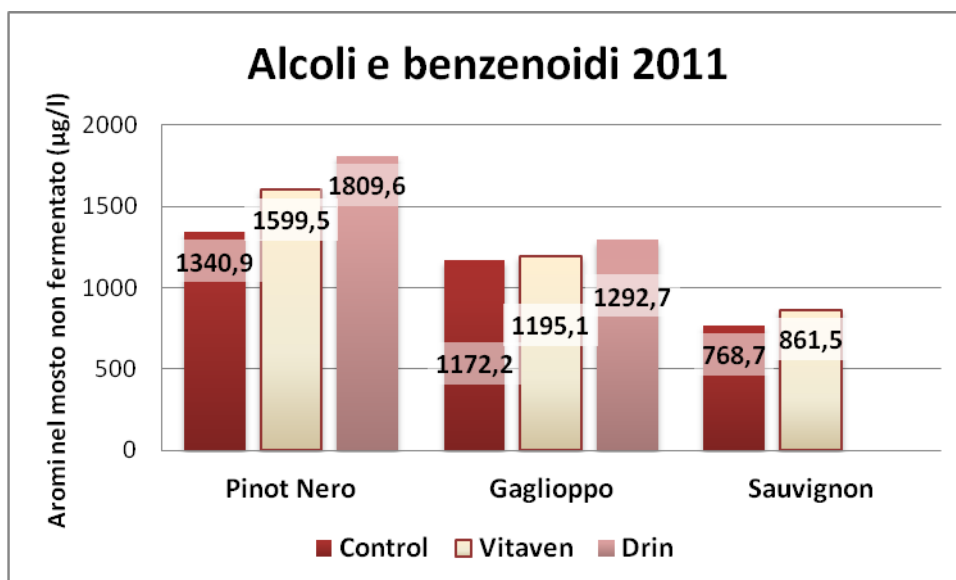
Graf.4: risultati del contenuto in alcoli e benzenoidi in mosto non fermentato Pinot nero, Gaglioppo and Sauvignon_2011.
