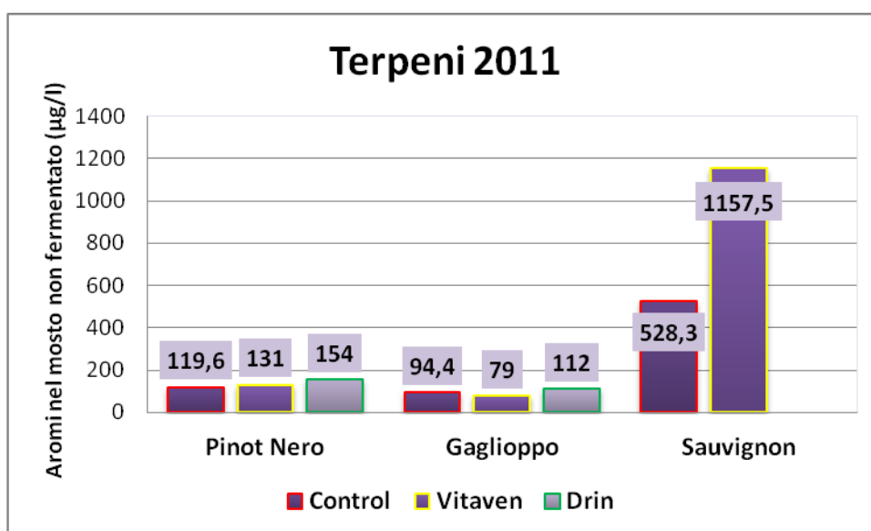
Graf.5: risultati del contenuto in terpeni in mosto non fermentato Pinot nero, Gaglioppo and Sauvignon_2011.
