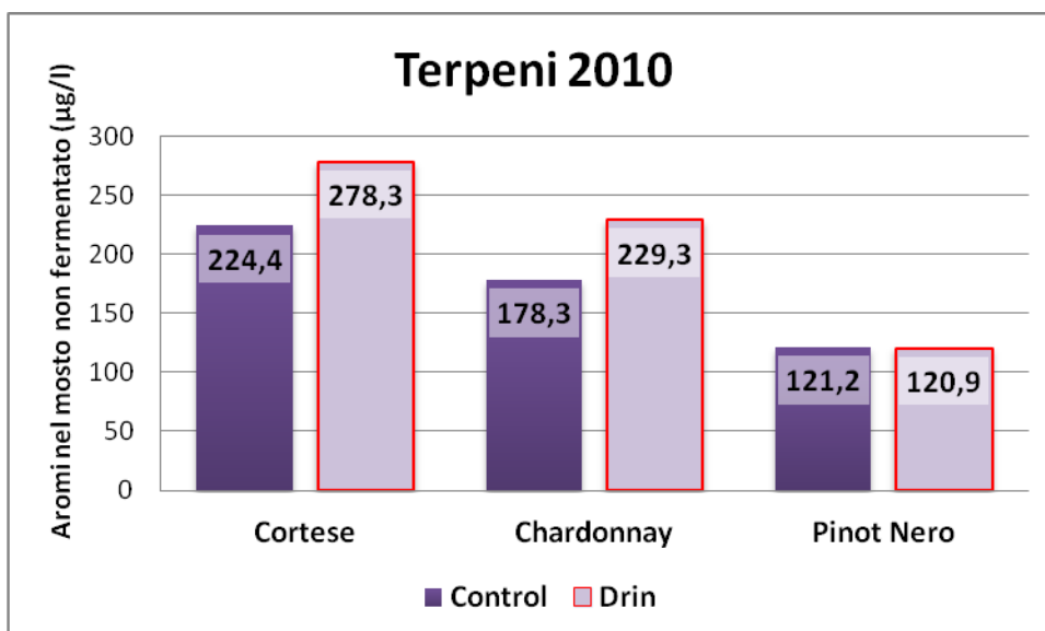
Graf.2: risultati del contenuto in terpeni in mosto non fermentato di Cortese , Chardonnay e Pinot Nero _2010.
