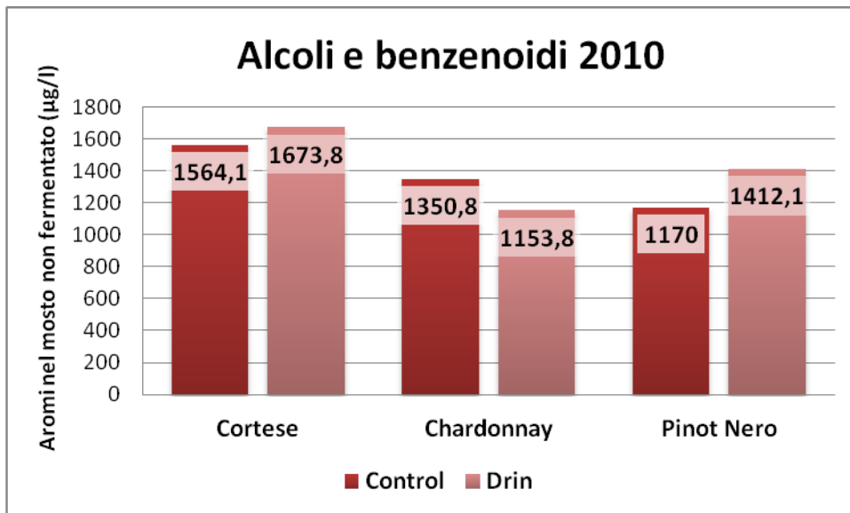
Graf.1: risultati del contenuto in alcoli e benzenoidi in mosto non fermentato di Cortese , Chardonnay e Pinot Nero _2010.
