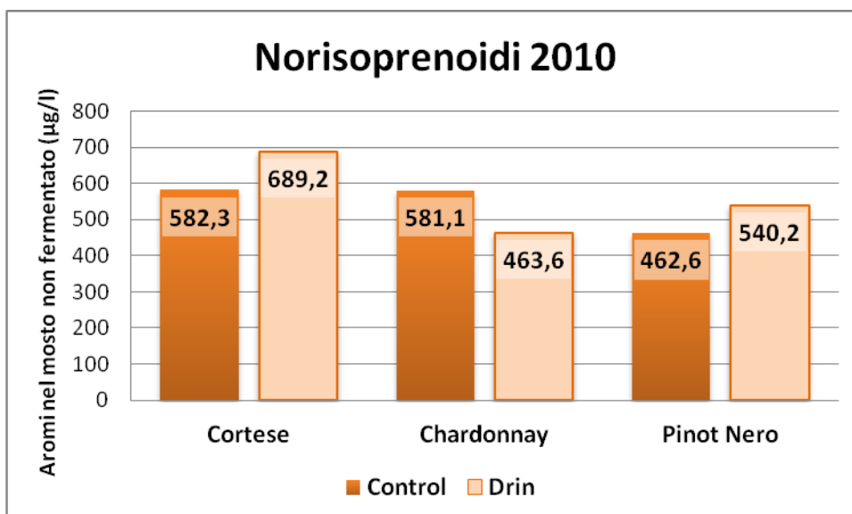
Graf.3: risultati del contenuto in norisoprenoidi in mosto non fermentato di Cortese , Chardonnay e Pinot Nero _2010.
