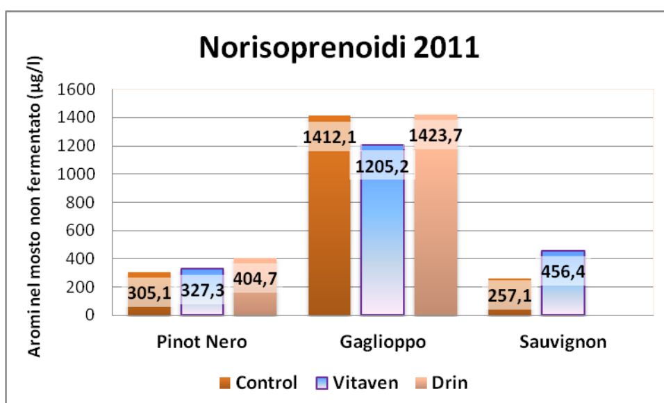
Graf.6: risultati del contenuto in norisoprenoidi in mosto non fermentato Pinot nero, Gaglioppo and Sauvignon_2011.
